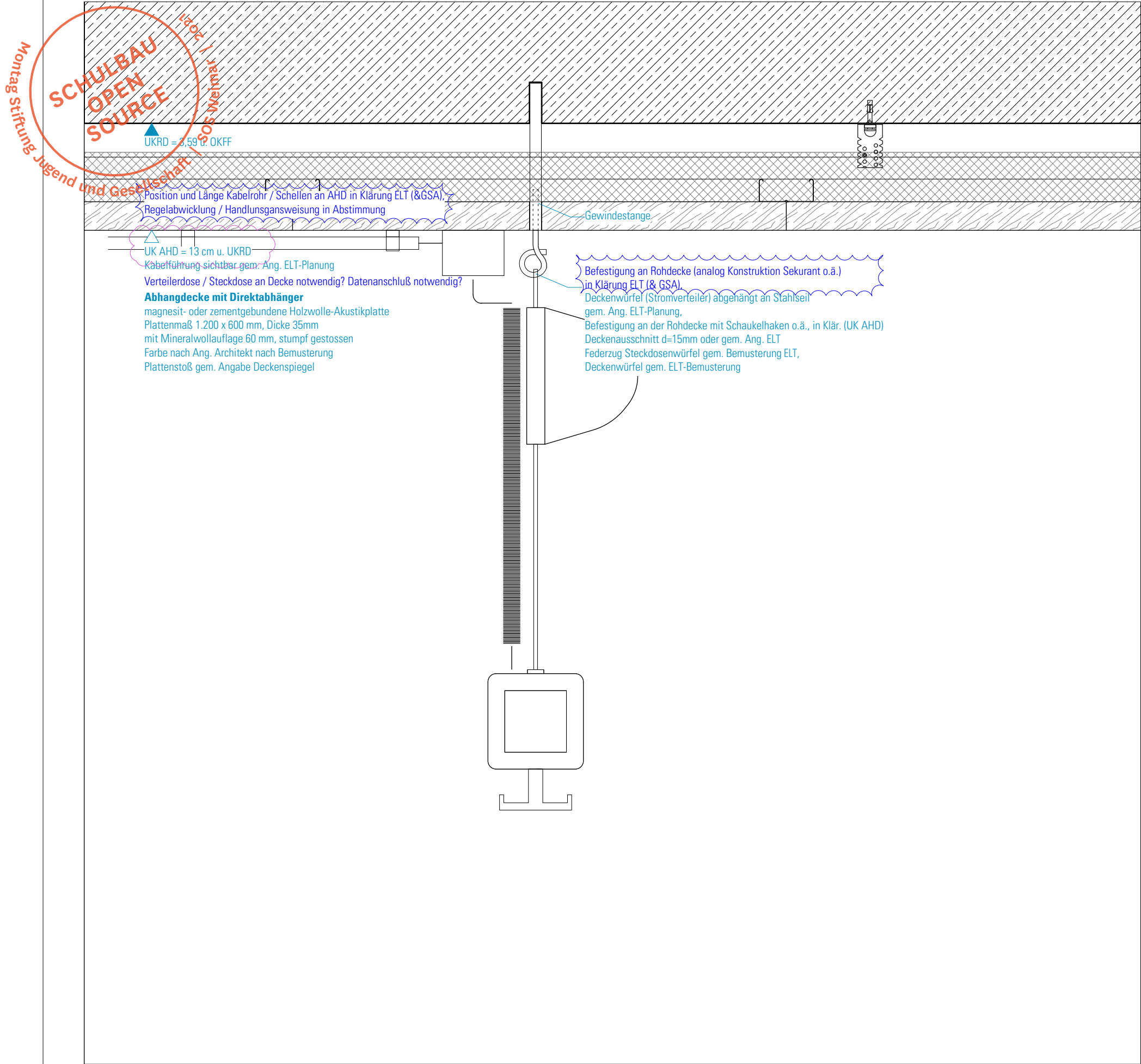
Detail Deckenwürfel
