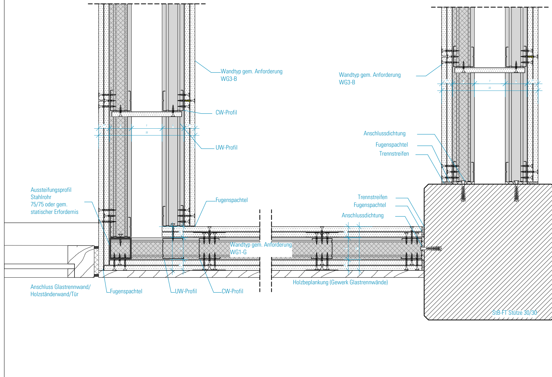
F60-Anschlüsse Stütze/Glastrennwand/Ecke
