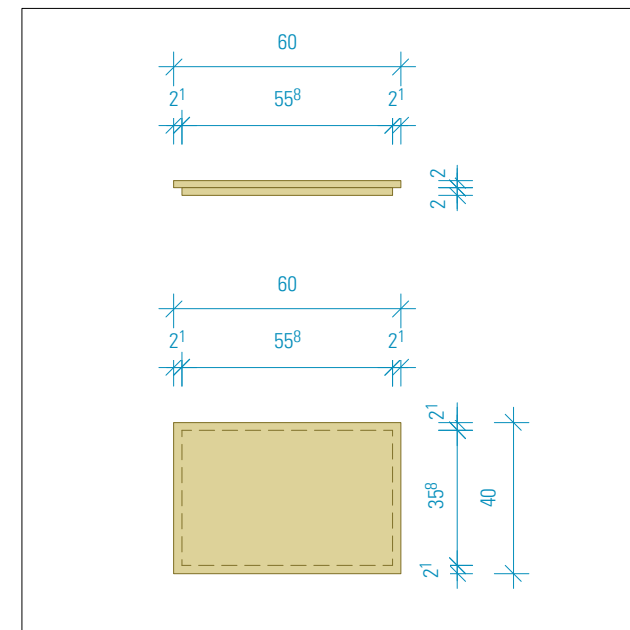
Deckel für Euroboxen 600 x 400 mm
